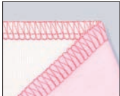
4本糸縁かがり
