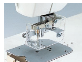
ニードルパンチアタッチメント
